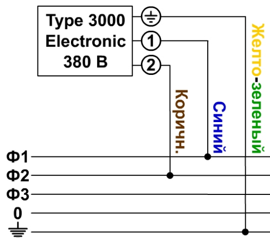
Рис.3 Коммутация к сети питания 380 В
