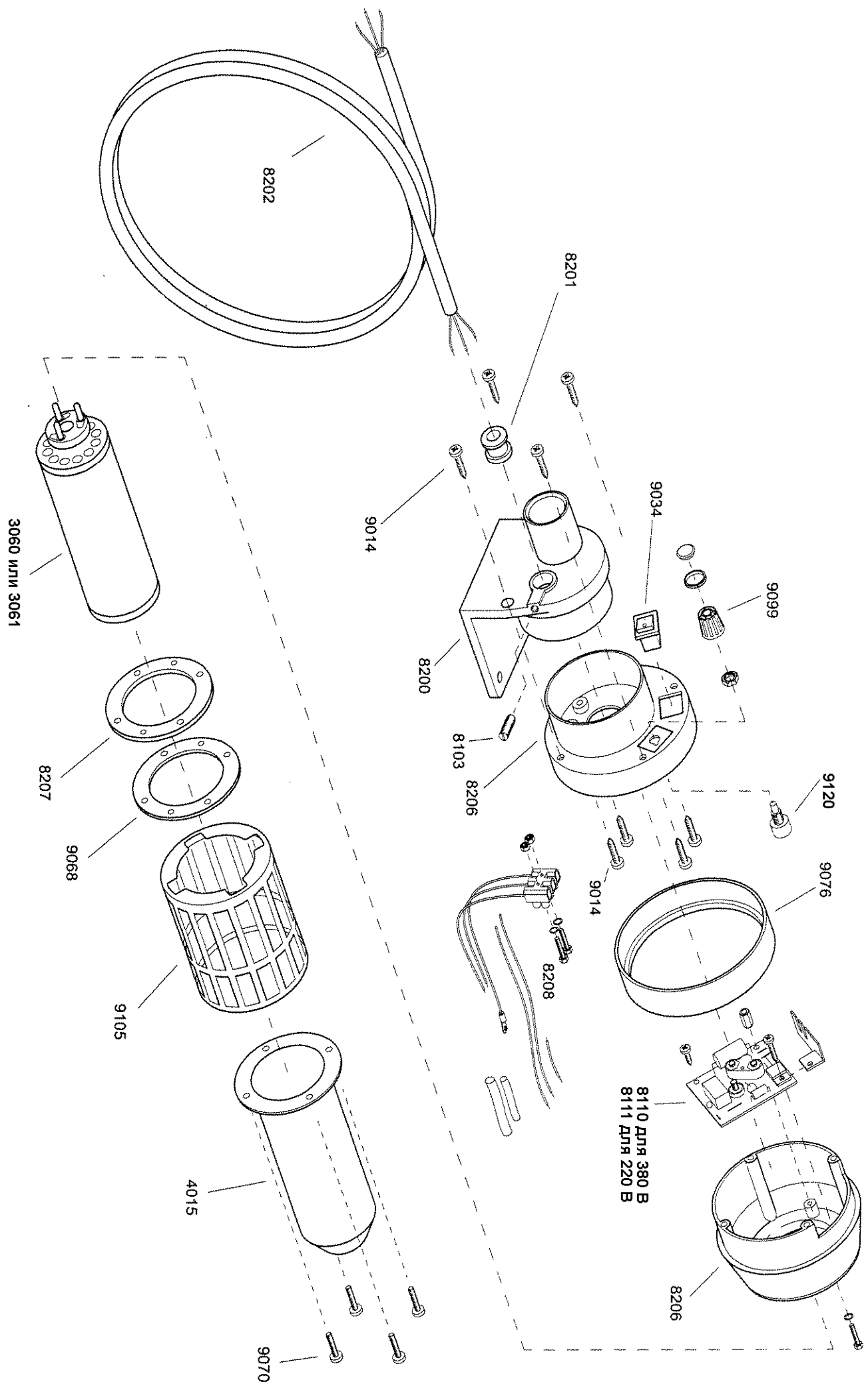
Рис. 6 Сборочный чертёж промышленных нагревателей Типе 3000 Electronic
