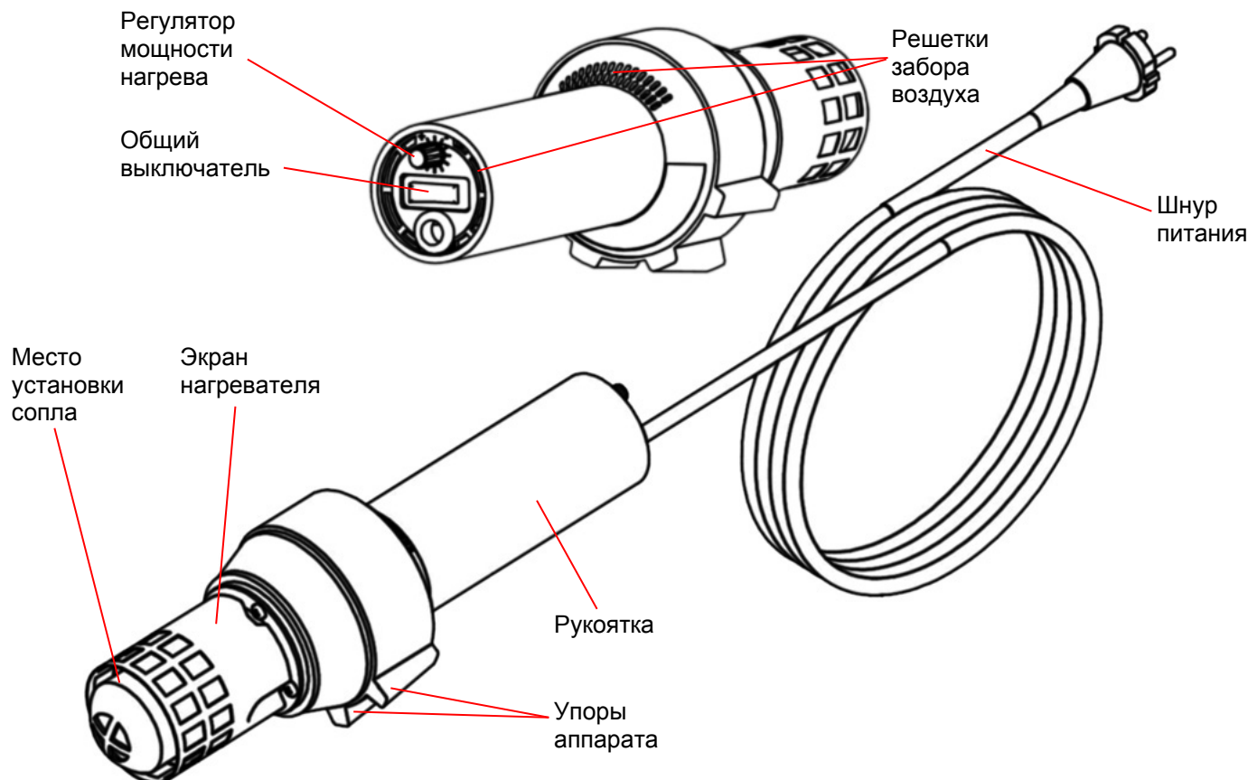
Рис. 2 Органы управления аппарата TUBE-Grand
