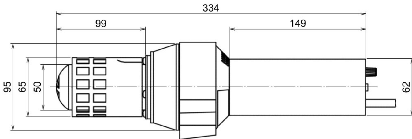
Рис. 1 Размеры аппарата TUBE-Grand
